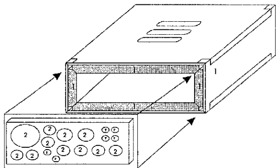
Rauchgasabdichtung aus 1,5 mm Styrolux
