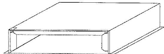
Bauart 4, dreiseitig, für einseitigen Bodenanschluss - Breite bis 435 mm - Höhe bis 80 mm - Tiefe 270 mm - mit und ohne Bodenblech
