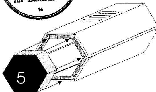
Rauchgasabdichtung aus 4 cm dicken "EasyFoam - Schaumstopfen"
