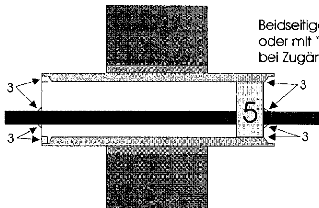
Rauchgasabdichtung aus 1,5 mm Styrolux
